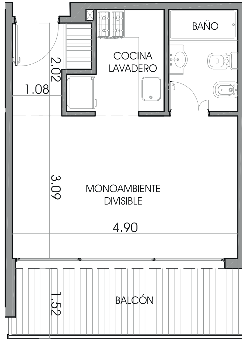
PLANTA DE LA UNIDAD
