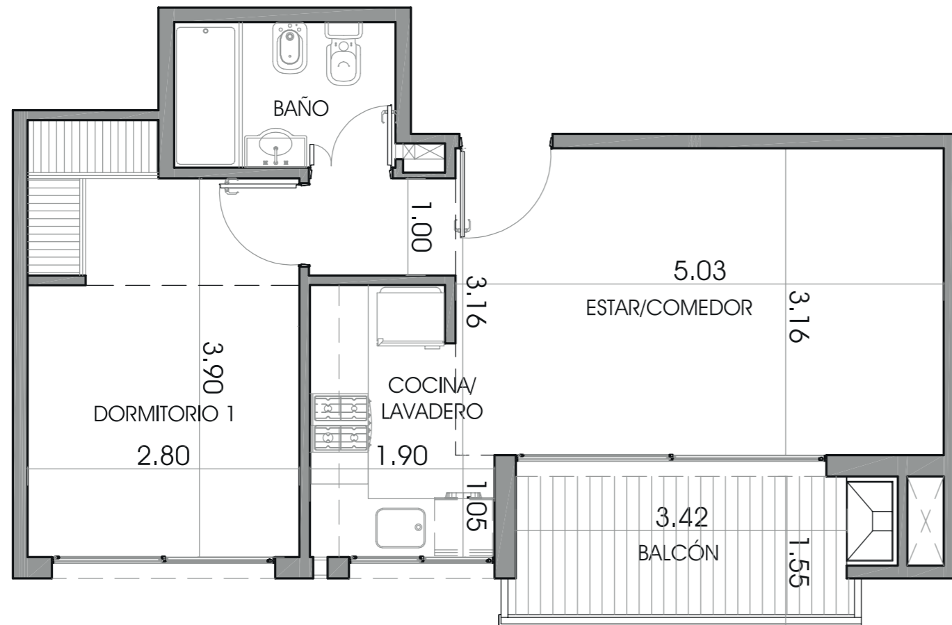
PLANTA DE LA UNIDAD
